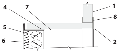
Metszeti rajz
