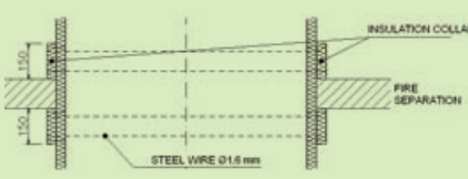
Tűzmegállítási kör keresztmetszetű vezeték esetén
