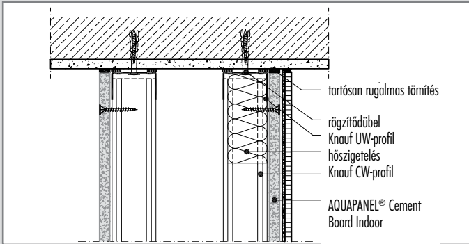
W386-V01 Mennyezet csatlakozás
