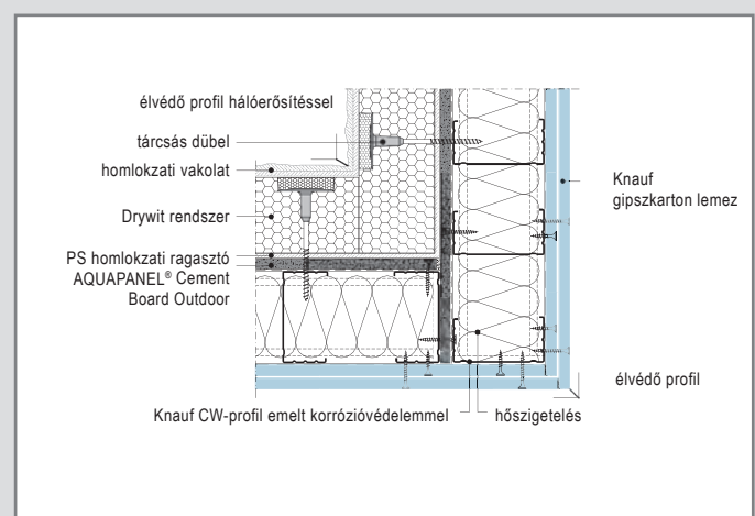
W384E-VM-ETICS1 Negatív sarok
