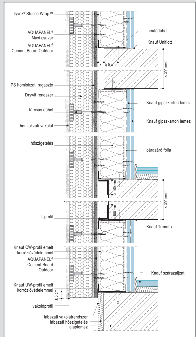
W384E-V-ETICS1 Metszet
