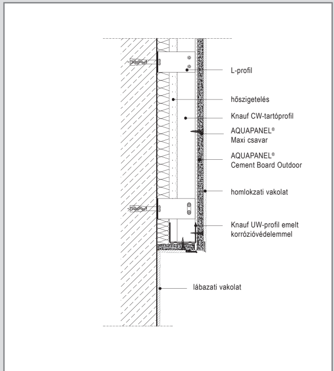
W684T-SO-V2 Lábazat kialakítás
