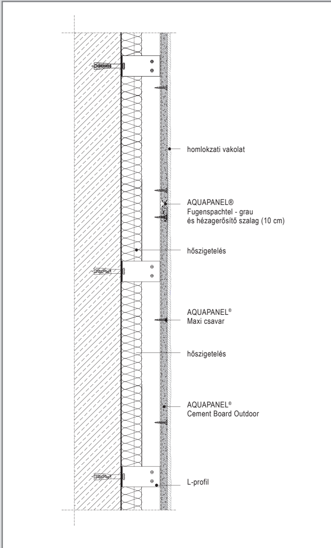
W684T-V1 Metszet
